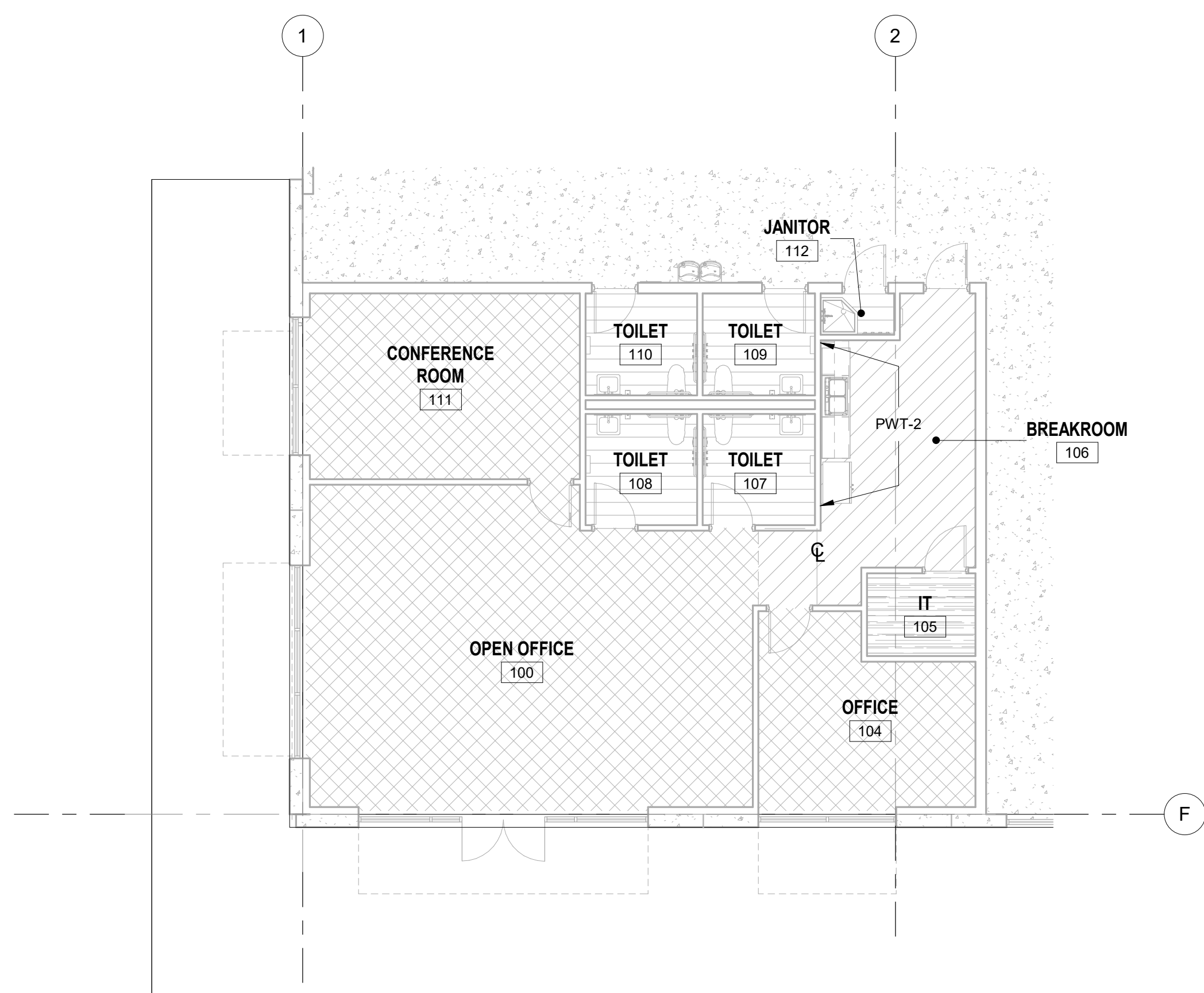
D1 FINISH PLAN - OFFICE SCALE: 1/8" = 1'-0"
